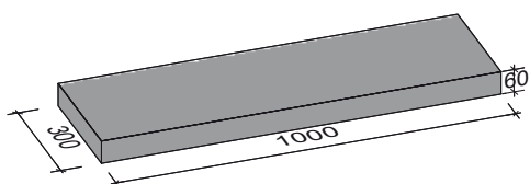
Mauerabdeckung Kopf
